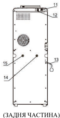
Мал.1: Схема апарата СН-V118En
